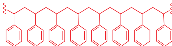
聚苯乙烯结构一个片段
