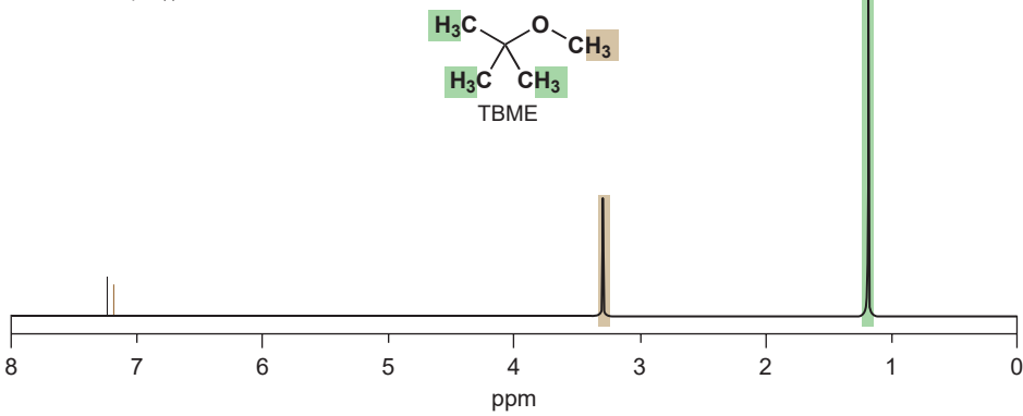
1 H NMR 光谱
