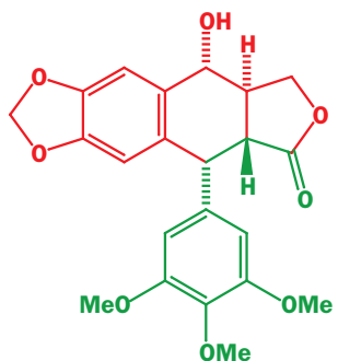
鬼臼毒素
