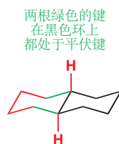
反-十氢化萘
