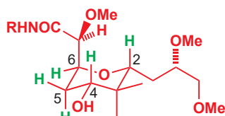
隐翅毒素右侧环的构象
