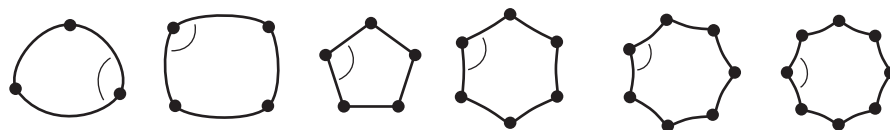
所有内角均为 109.5^\circ
