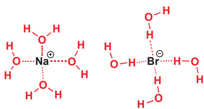
水可以溶剂化阳离子和阴离子
