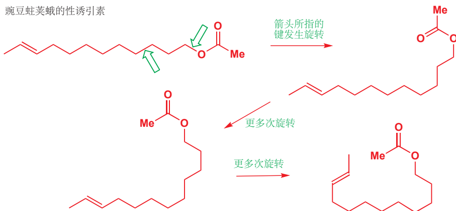
豌豆蚜的性诱引素
