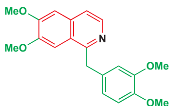
罂粟碱——一种苜蓿异喹啉生物碱
