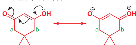
双甲酮烯醇式中的离域
