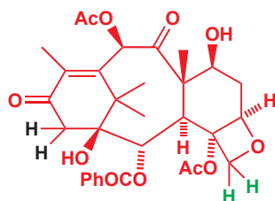
隐翅毒素右侧环的构象
