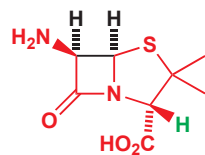
青霉烷酸 (penicillanic acid)
