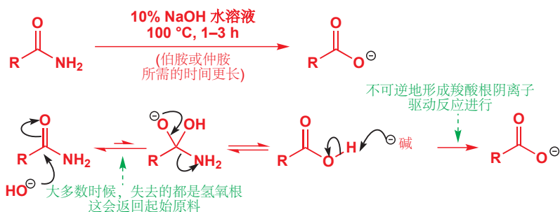
碱性下的酰胺水解
