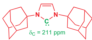
一种稳定的 N-杂环卡宾
