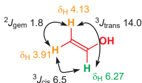
乙烯醇的 NMR 光谱
