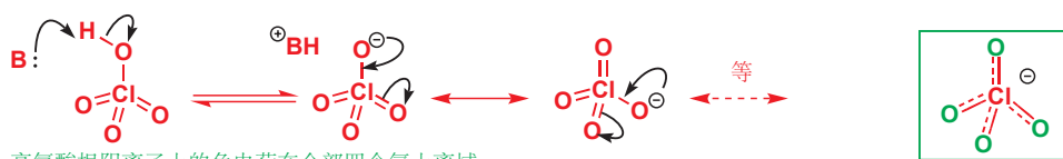
高氯酸根阴离子上的负电荷在全部四个氧上离域
