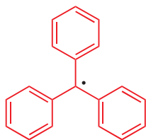
三苯甲基自由基— 在溶液中稳定 与其二聚体处于平衡
