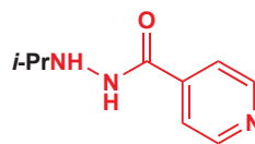
异丙烟肼 iproniazid
