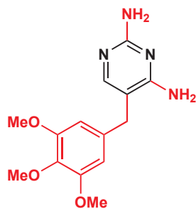
甲氧苄氨嘧啶
