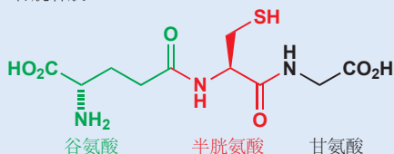
谷胱甘肽
