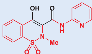
Piroxicam (Feldene®) 治疗关节炎 每日一次
