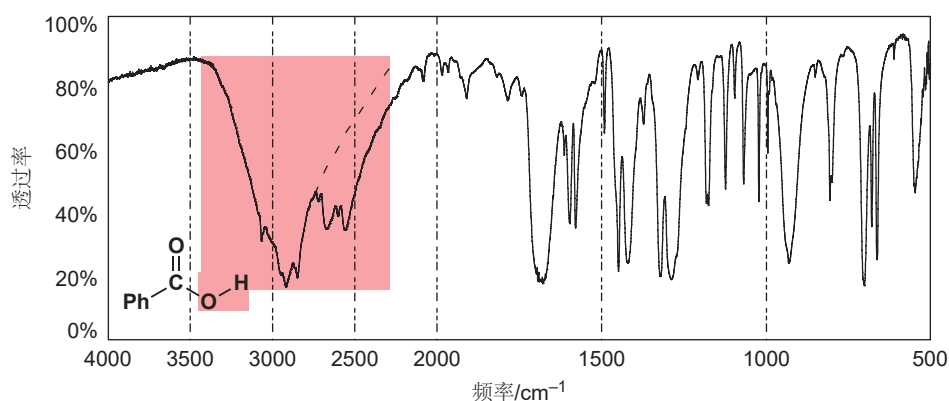
光谱 4
