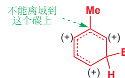
间位取代的不利中间图
