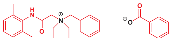
“苯甲地那铵 (denatonium benzoate)”，苦精 (Bitrex) 苯甲酸 苄基二乙基[(2,6-二甲苯基氨基甲酰基)甲基]铵
