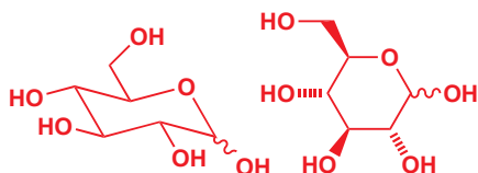
葡萄糖的两种表达方式
