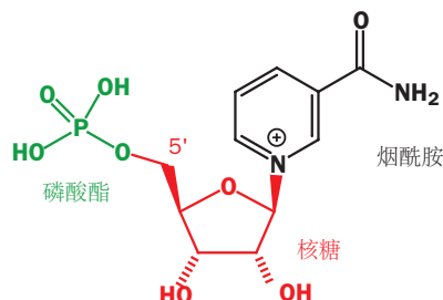
一种烟酰胺核苷酸
