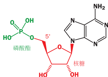
AMP——一种腺嘌呤核苷酸
