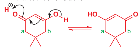
双甲酮烯醇式中的互变异构
