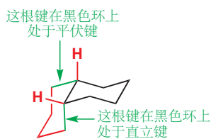
顺-十氢化萘
