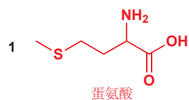
蛋氨酸
