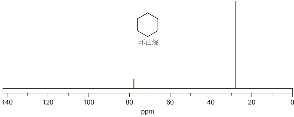
13 C NMR 光谱
