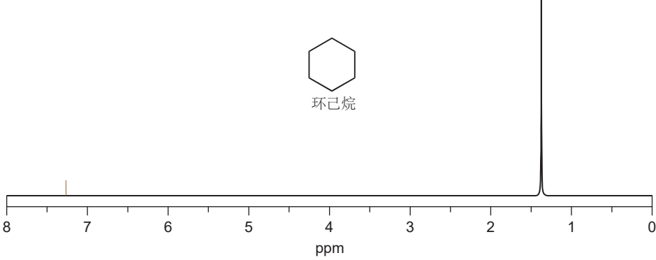
1 H NMR 光谱
