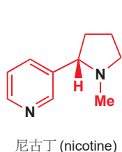
尼古丁 (nicotine)
