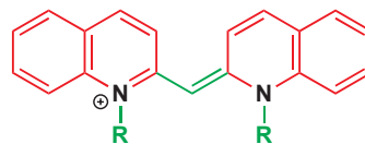
一种“花青色”染料
