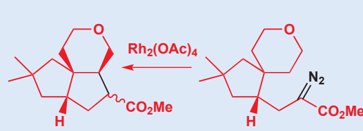
路线 2: Taber
