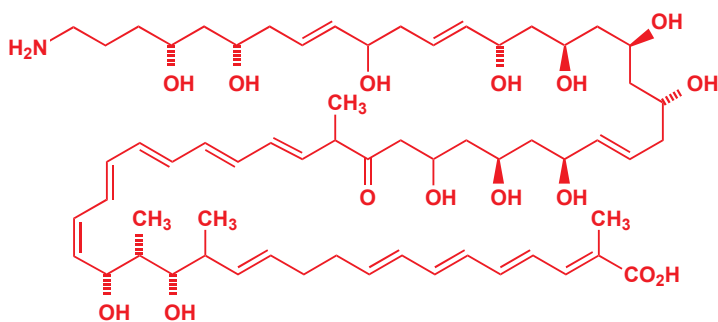
线性霉素
