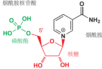
烟酰胺核苷酸
