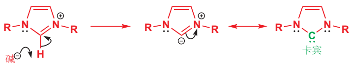
咪唑鎓阳离子的去质子得到卡宾
