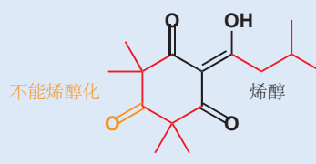
Leptosperme (Callisto®) 瓶刷状植物美花红千层生产的除草剂
