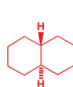
反-十氢化萘
