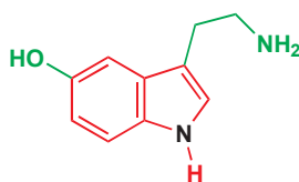
血清素—— 一种神经递质
