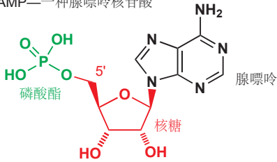
AMP——一种腺嘌呤核苷酸
