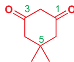
“双甲酮 (dimedone)” 5,5-二甲基-1,3-环己二酮
