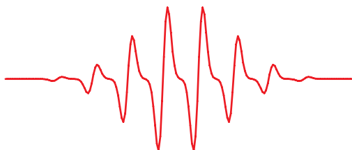
环庚三烯基自由基的 ESR 光谱
