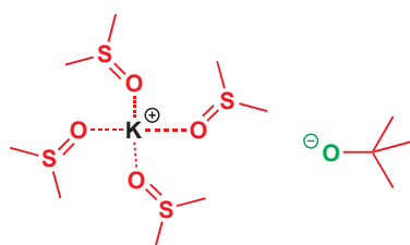
DMSO (非质子极性溶剂) 只能溶剂化阳离子
