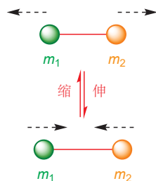
红外中键的振动
