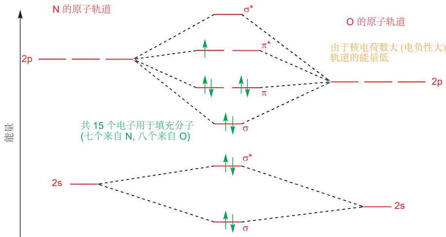
一氧化碳 (NO) 的分子轨道图 (1s 轨道已省略)
