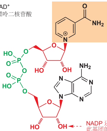
\text{NAD}^+ 及 \text{NADP} 的活性部分
