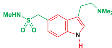
舒马普坦：治疗偏头痛
