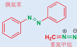
偶氮苯
