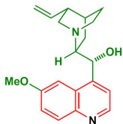
奎宁
