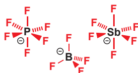
非亲核性阴离子
