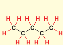
链 (chain)
