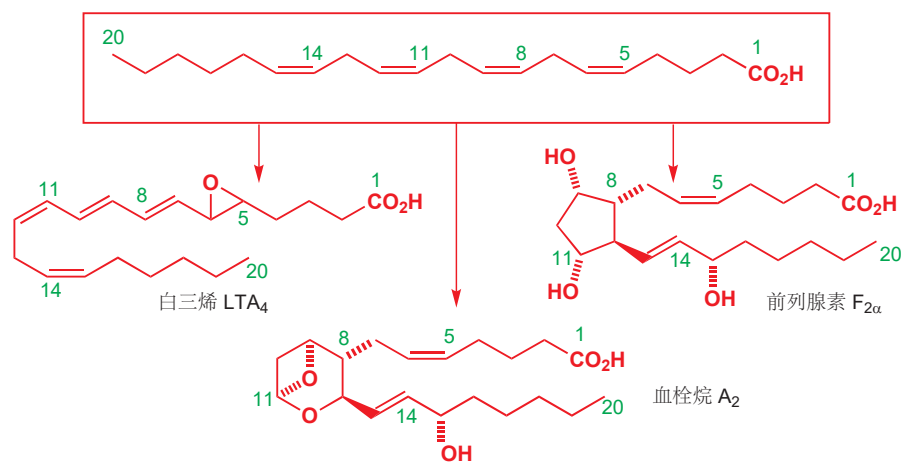
由花生四烯酸合成的化合物
