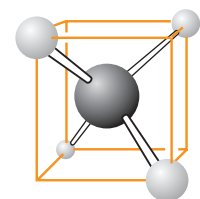
立方体中的甲烷分子
