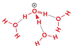
水中溶剂化的水合氢离子/水合氢离子 (hydronium ion) 的结构: 虚线表示氢键
